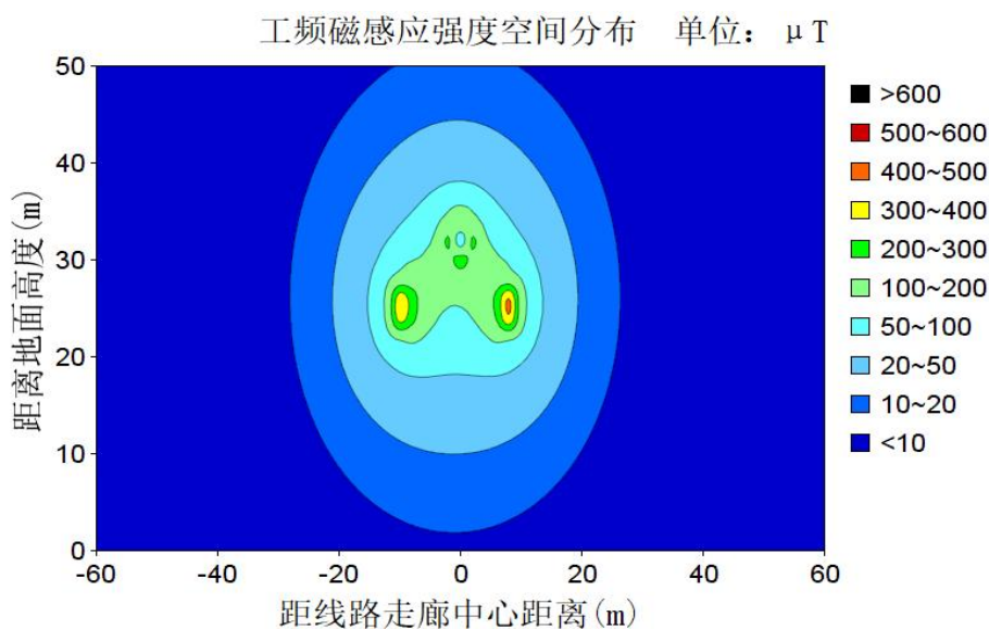
图 6-4 500kV 广山一线新建段磁感应强度空间分布图
