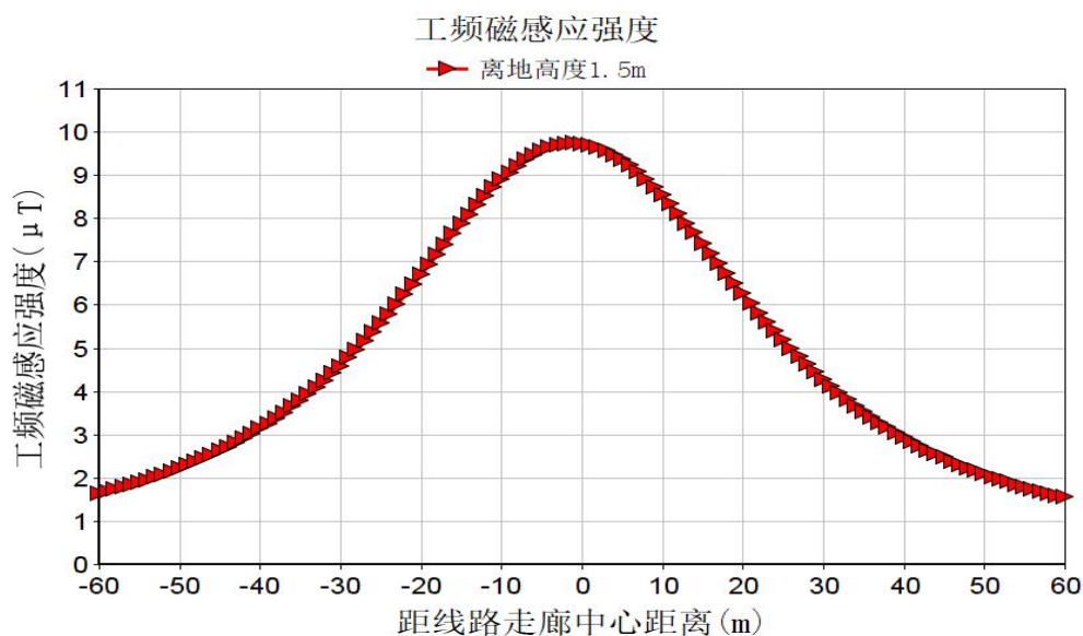
图 6-3 500kV 广山一线新建段地面 1.5m 高处磁感应强度分布曲线图
