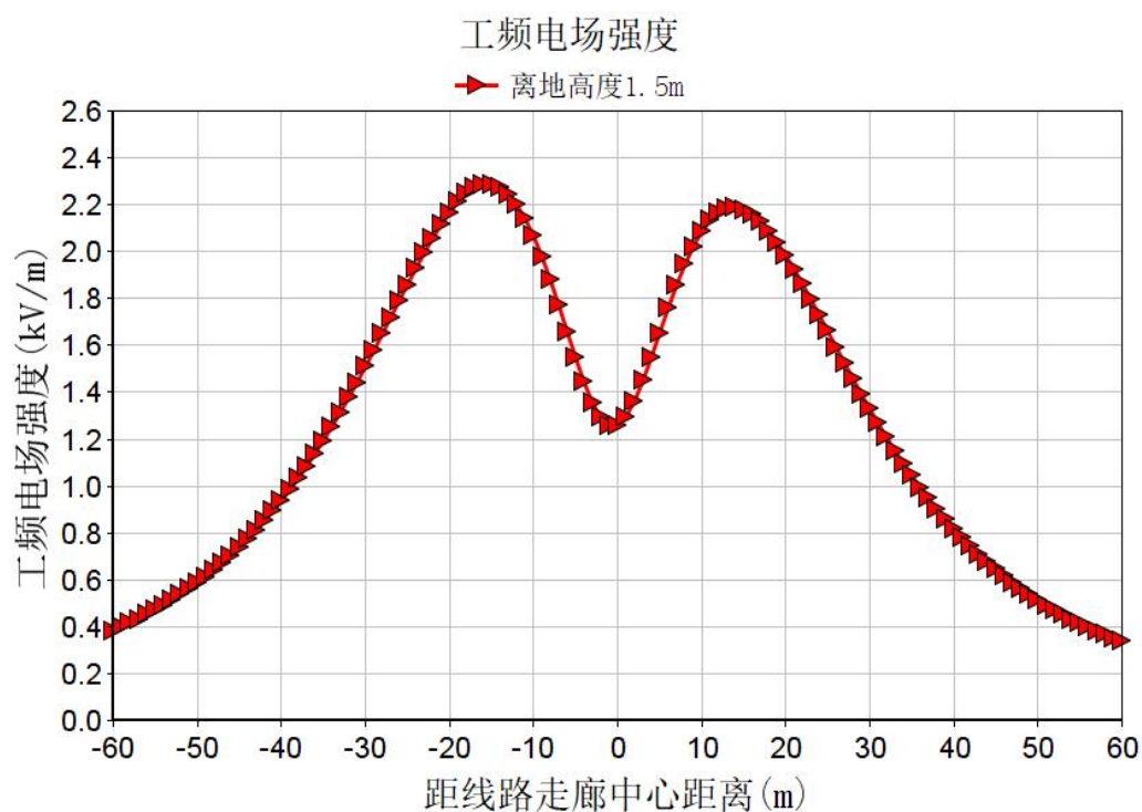
图 6-1 500kV 广山一线新建段地面 1.5m 高处电场强度分布曲线图
