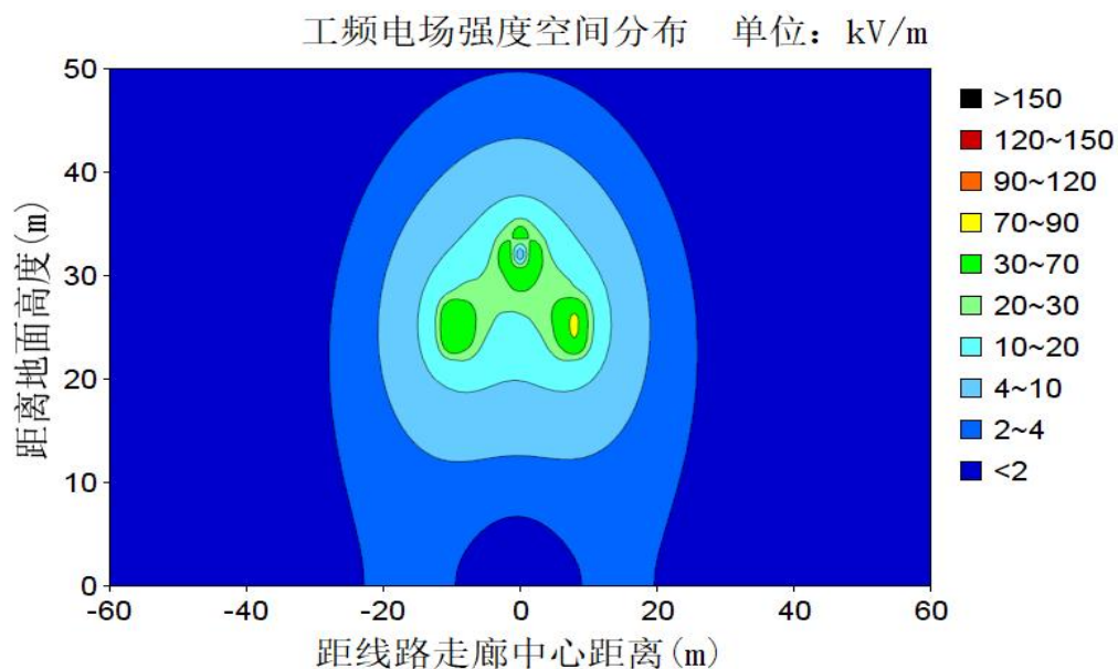
图 6-2 500kV 广山一线新建段电场强度空间分布图
